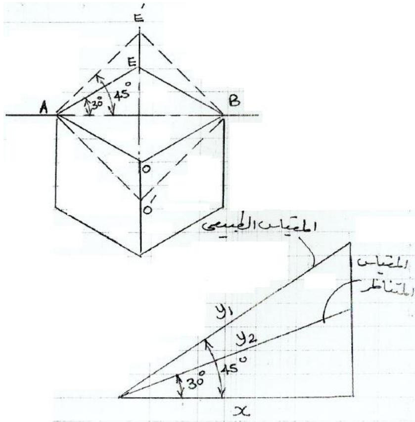
شكل (6.3) أسلوب أخذ الأبعاد في الإسقاط المتناظر
