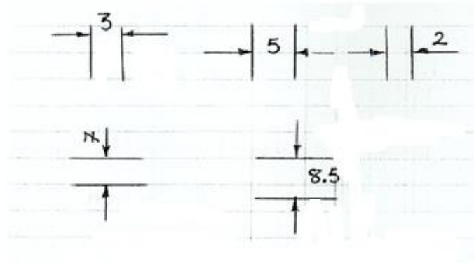
شكل (5.3) الأبعاد على الملامح الصغيرة (Dimensioning of small features)
