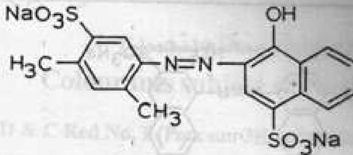
شكل (٢٩) FD&C Red No.4
