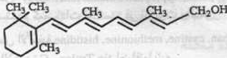
شكل (٢٣) Vitamin A
