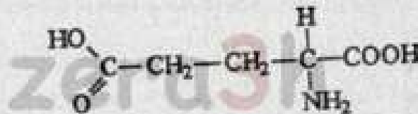
شكل (٩٤) تركيب MSG
