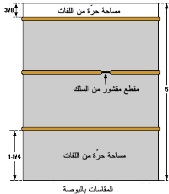
الوشيجة الأولى: لّف السلك حول الأنبوب
