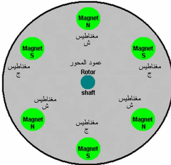
Rotor (1 required) دوّار (مطلوب واحد)
