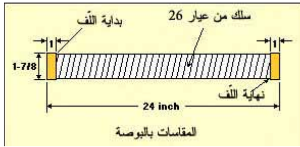
الوشيعّة الثانويّة
